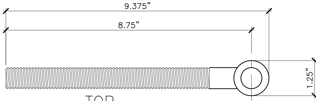
TOP
