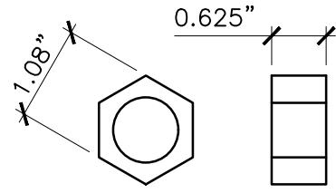
NUT X2
